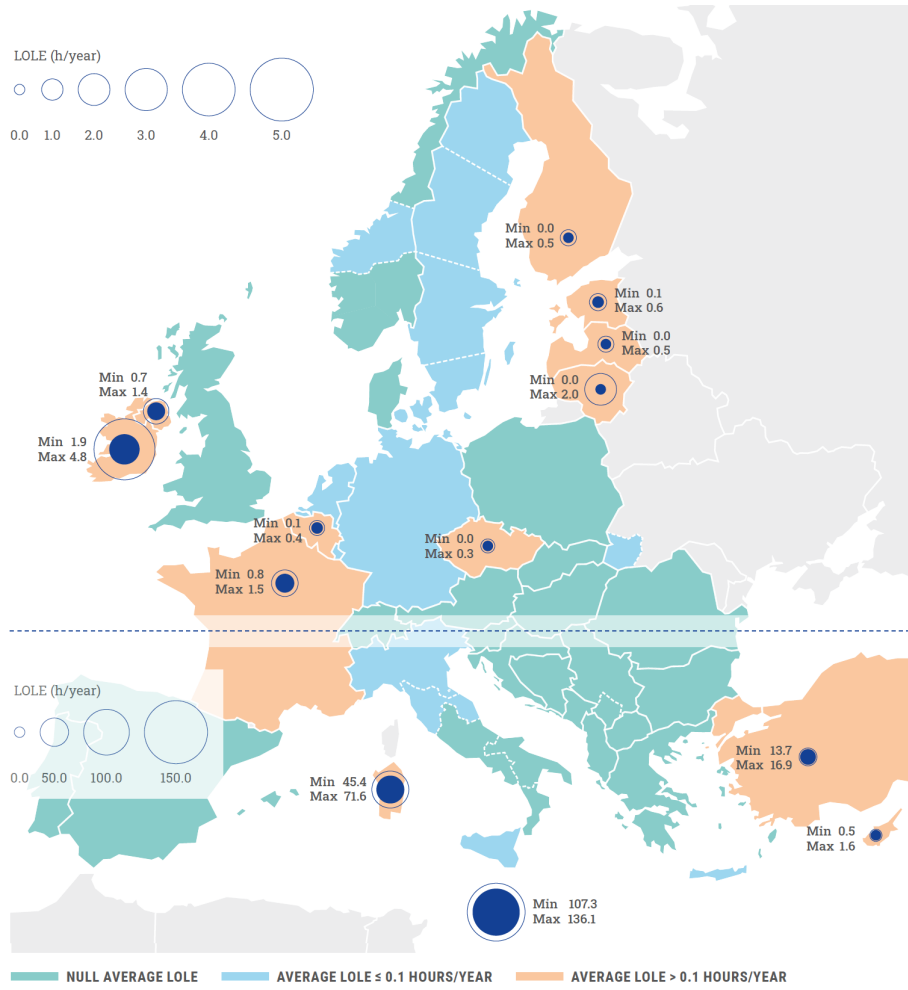
Abbildung 1 Mid-Term Adequacy Forecast für 2025: Ergebnisse LOLE, Bildquelle: (ENTSO-E, 2020)
