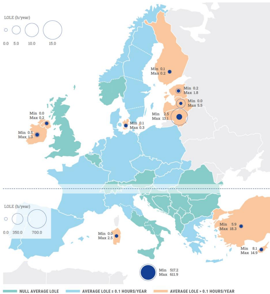
Abbildung 2 Mid-Term Adequacy Forecast für 2030: Ergebnisse LOLE, Bildquelle: (ENTSO-E, 2020)
