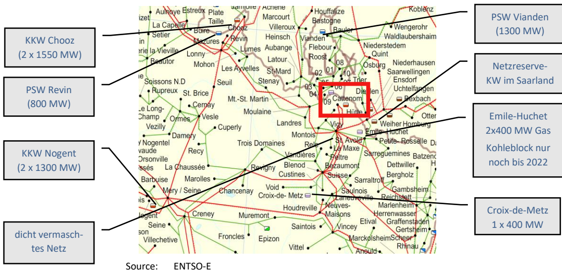
Abbildung 6 Übertragungsnetz und steuerbare Erzeugung in der Region (Bildquelle der Karte: ENTSO-E Grid Map, (ENTSO-E, o. J.)
