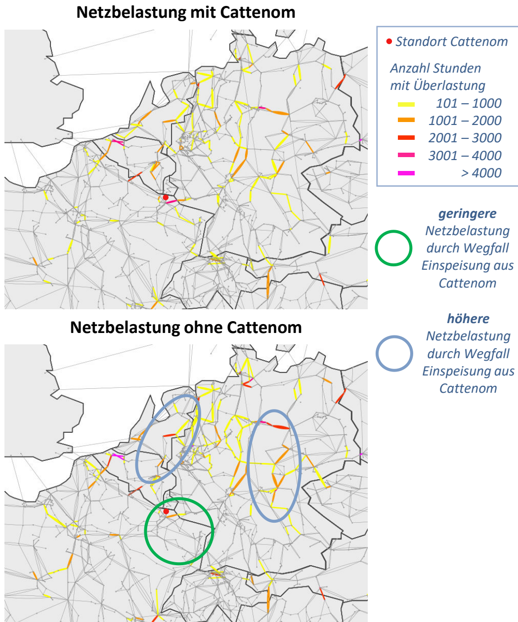
Abbildung 5 Entwicklung der Netzbelastung bis 2026 mit und ohne Weiterbetrieb des Kraftwerks Cattenom (eigene Berechnungen)
