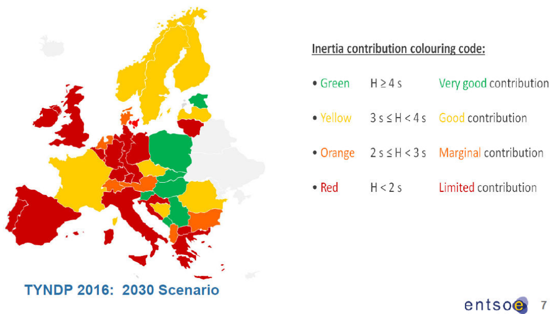
Abbildung 7 Trägheit im Synchronverbund Continental Europe 2030, Bildquelle (Mario Ndreko und ENTSO-E Technical Group on High Penetration, 2020)
